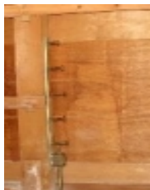
ホールダウンの金具の取り付け。
